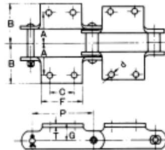
K2 附件尺寸图
