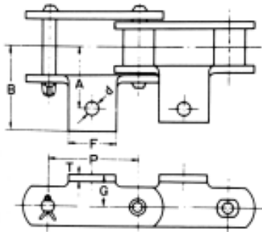
A1 附件尺寸图
