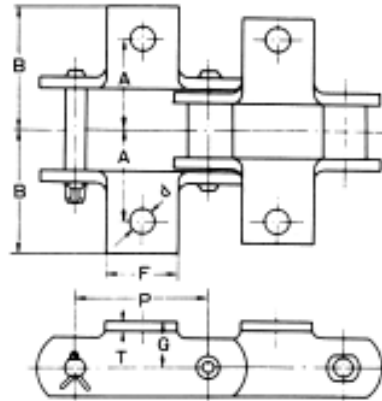
K1 附件尺寸图
