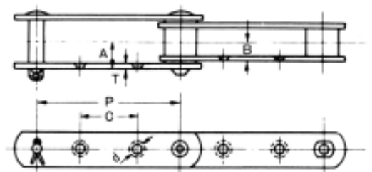
G2 附件尺寸图
