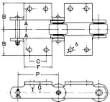
K2 附件尺寸图
