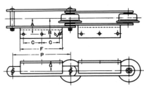
A3 附件尺寸图
