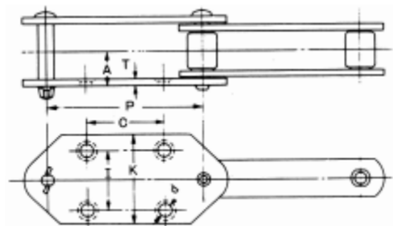
G4 附件尺寸图
