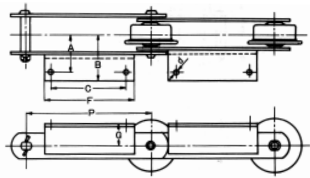
A2 附件尺寸图
