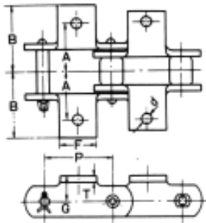
K1 附件尺寸图
