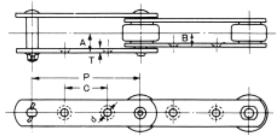
G2 附件尺寸图
