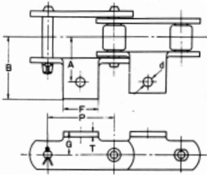
A1 附件尺寸图
