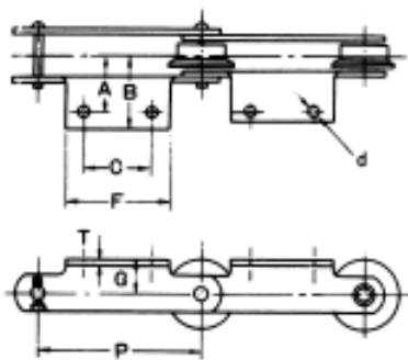
A2 附件尺寸图
