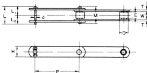
HRS 套筒式滚子链(S 型)尺寸图
