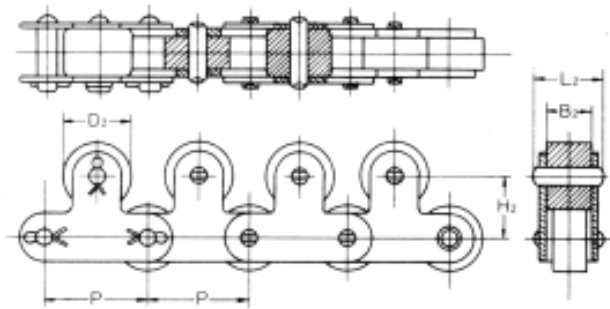
双节距顶端滚子链尺寸图
