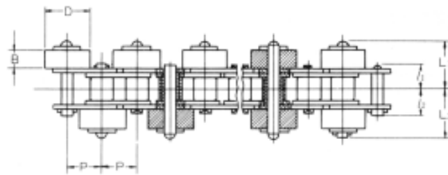
带有边滚轮的滚子链的尺寸图
