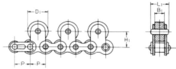
顶端滚子链尺寸图
