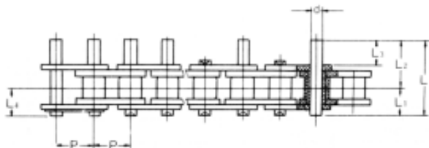
具有D式销轴的滚子链尺寸图
