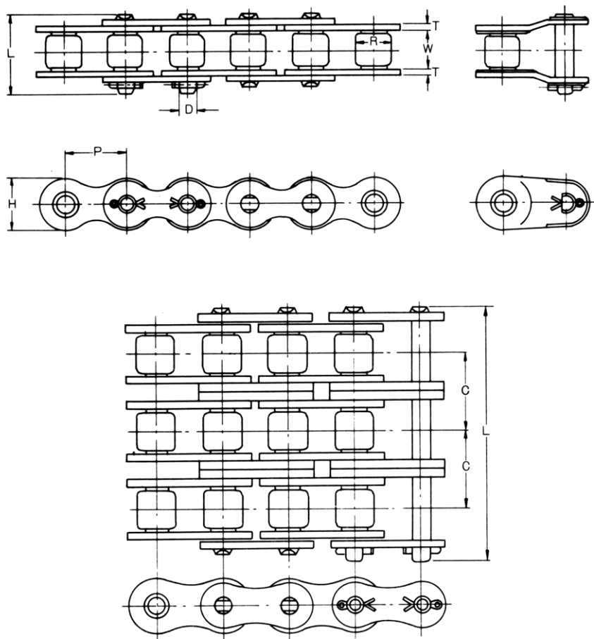
BS 链的尺寸图
