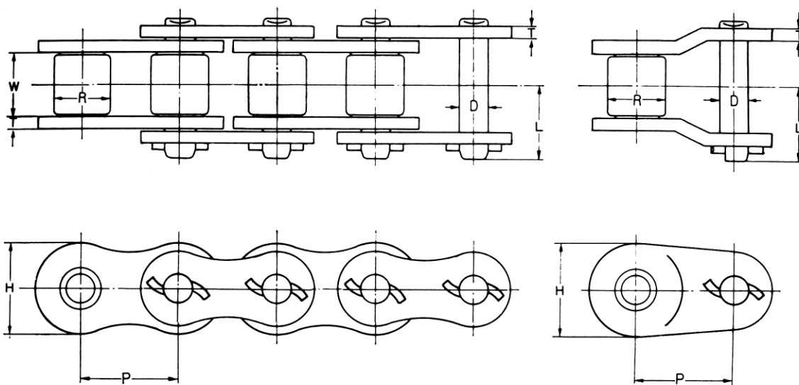
H 型滚子链条的尺寸图解
