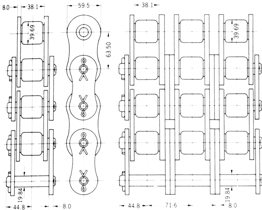
200号链条的尺寸
