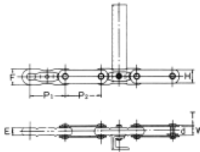
HBF 型谷仓清扫链的尺寸图
