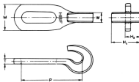
HBC 型谷仓清扫链的尺寸图
