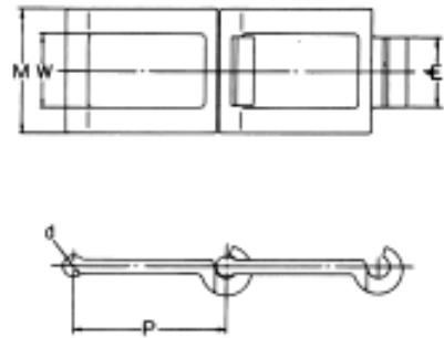
可拆卸钢链的尺寸与强度
