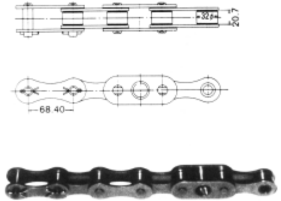
自动扶梯链的尺寸图
