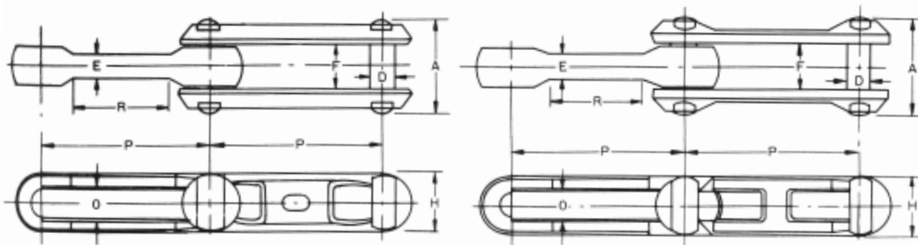
落锻链的尺寸与强度
