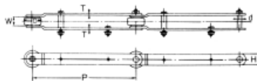
运输链的尺寸图
