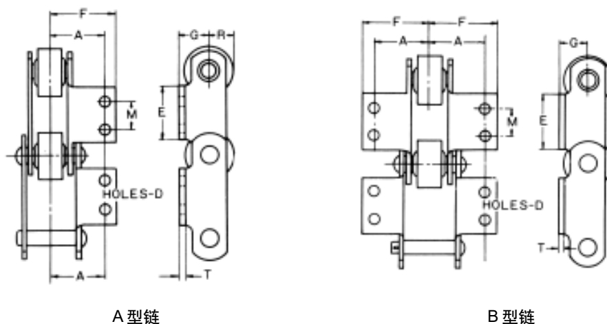
英式链的尺寸图
