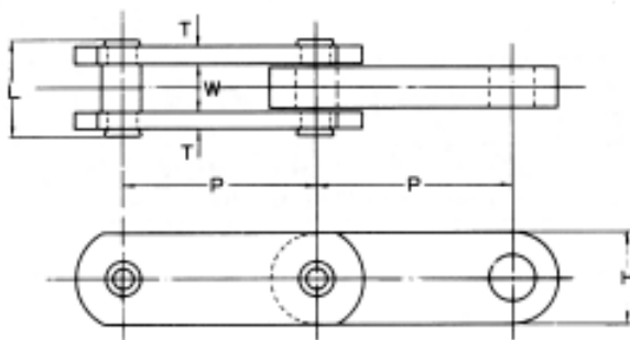
钢块输送链尺寸图
